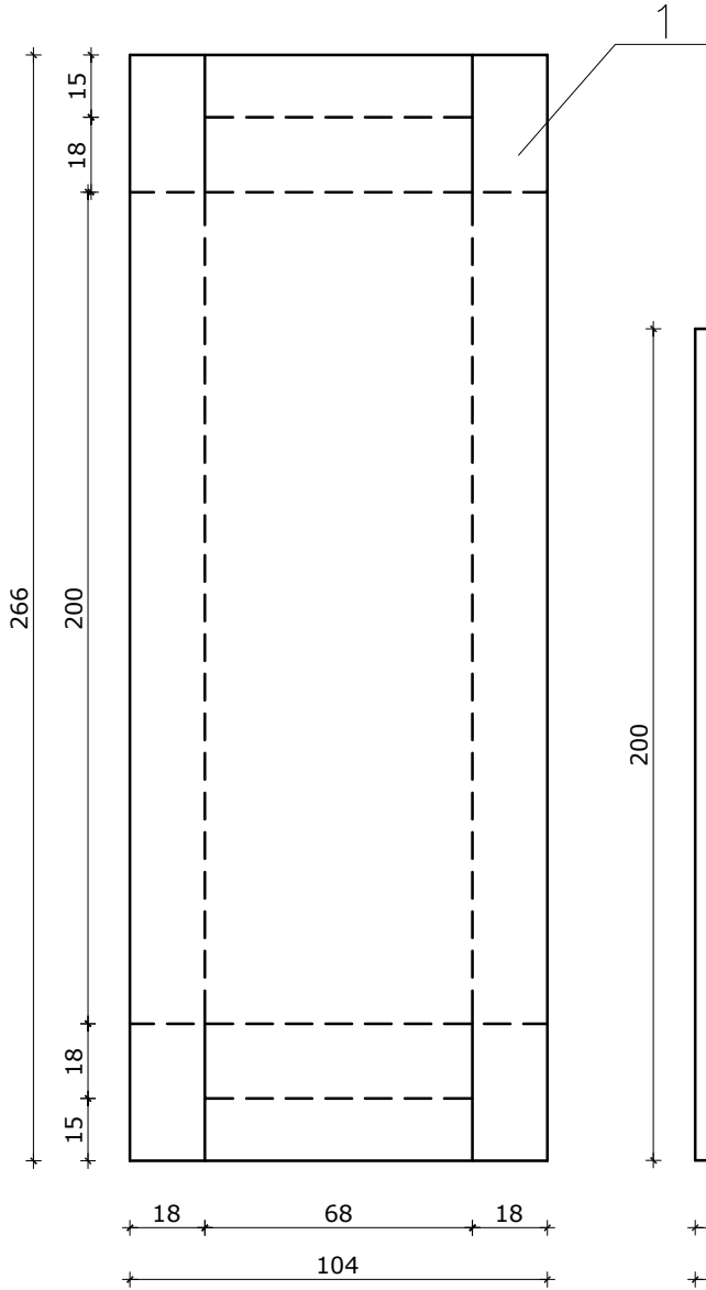
Детаљ савијања 1
